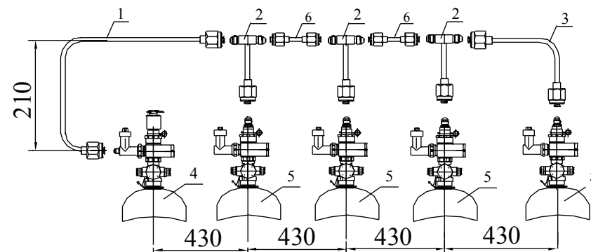
Схема монтажа КПП-4
