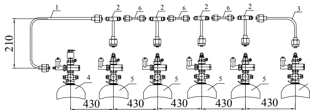
Схема монтажа КПП-5
